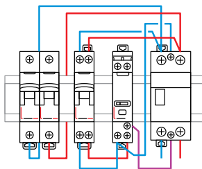
Spínanie jednofázového výkonového stykača.
