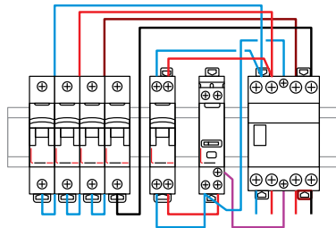
Spínanie trojfázového výkonového stykača.
